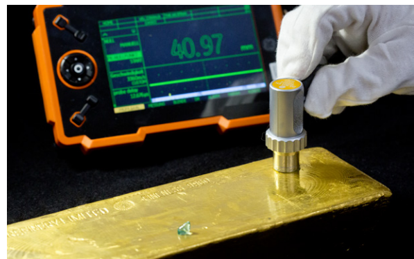
Ultraschallmessung.
